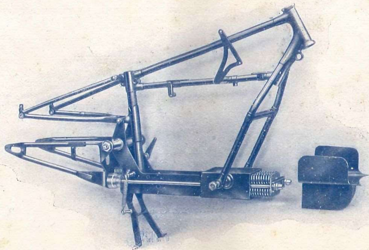
TELAIO ELASTICO - Brevettato.
