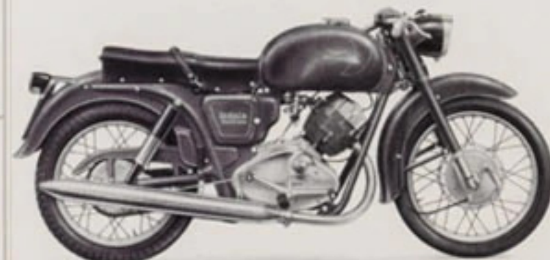
Modello/Anno: Lodola GT / 1956 Motore: Quattro Tempi Monocilindrico Inclinato 65 x 64mm /235cc Potenza: 11 CV a 6500 Giri/Min Peso: 115 Kg Velocità Massima: 115 KM/h
