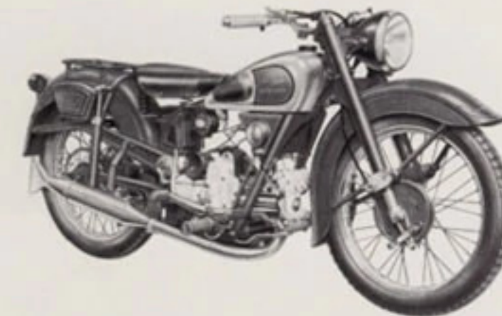
Modello/Anno: Airone / 1949 Motore: Quattro Tempi Monocilindrico Orizzontale 70 x 64mm /246cc Potenza: 9,5 CV a 4800 Giri/Min Peso: 142 Kg Velocità Massima: 95 KM/h
