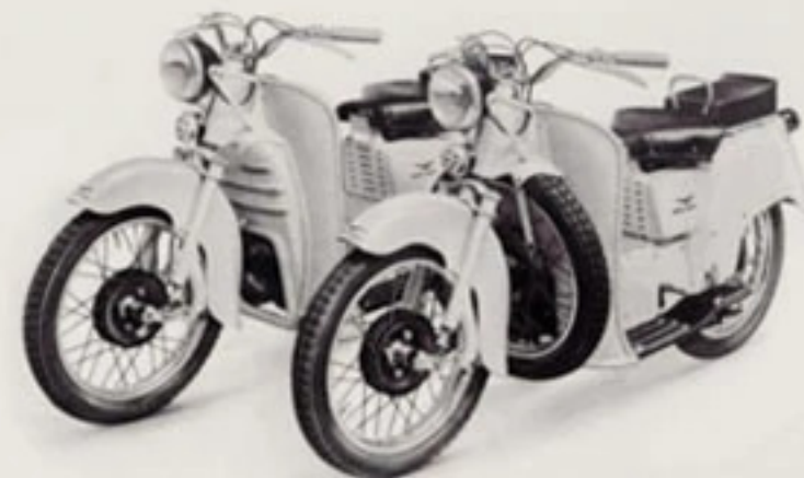
Modello/Anno: Galletto / 1950 - 1966 Motore: Quattro Tempi Monocilindrico Orizzontale 62 x 53mm /159,5cc Potenza: 6 CV a 5200 Giri/Min Peso: 107 Kg Velocità Massima: 50 KM/h
