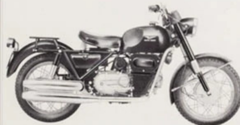
Modello/Anno: Nuovo Falcone Militare / 1965 Motore: Quattro Tempi Monocilindrico Orizzontale 55 x 52mm /498,4cc Potenza: 26,2 CV a 4800 Giri/Min Peso: a vuoto 214 Kg Velocità Massima: circa 127 KM/h
