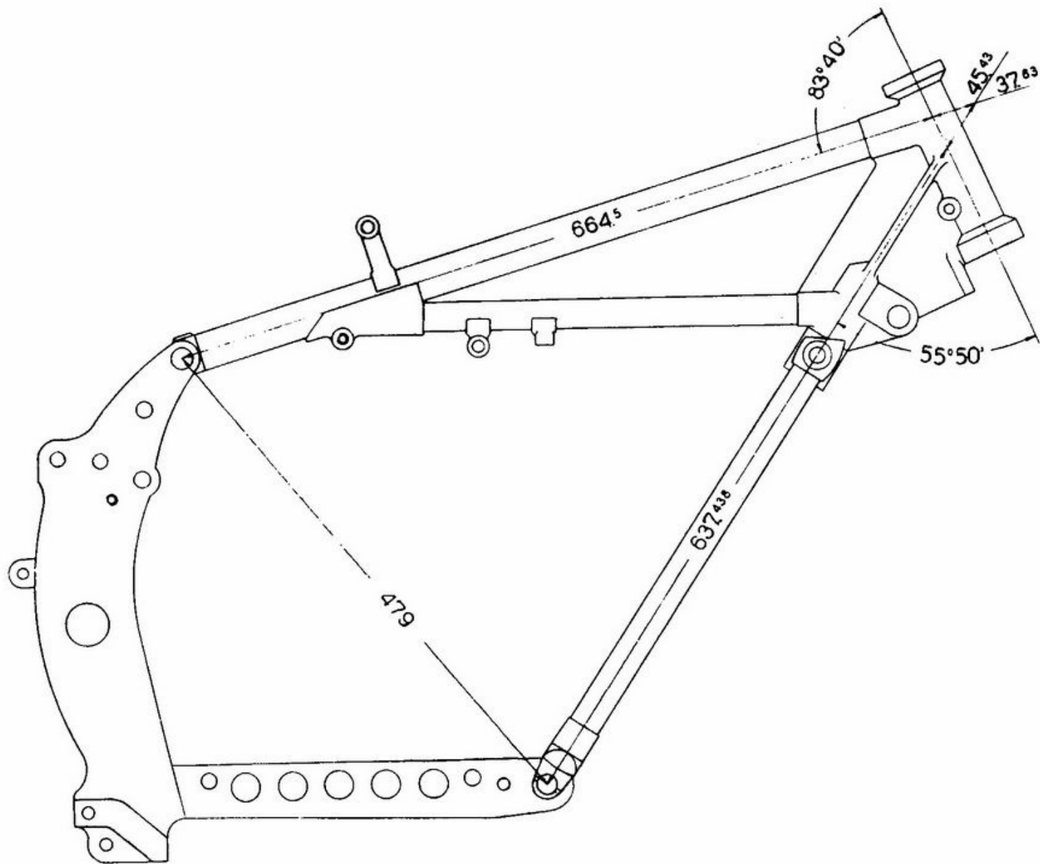
Fig. 34 - Telaio
