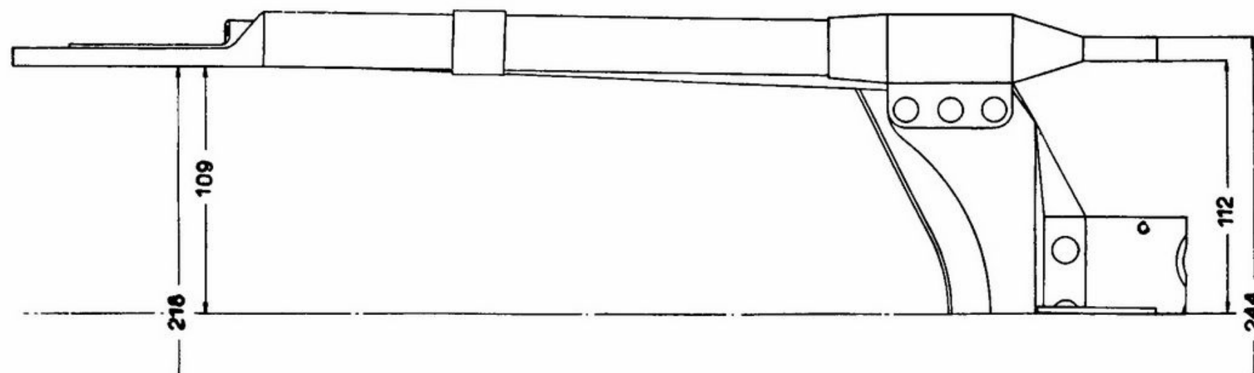
Fig. 35 - Forcellone oscillante
