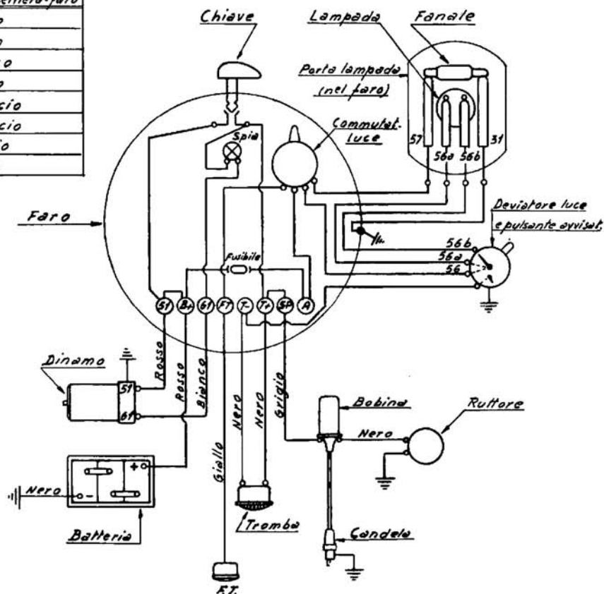
SCHEMA IMPIANTO ELETTRICO
