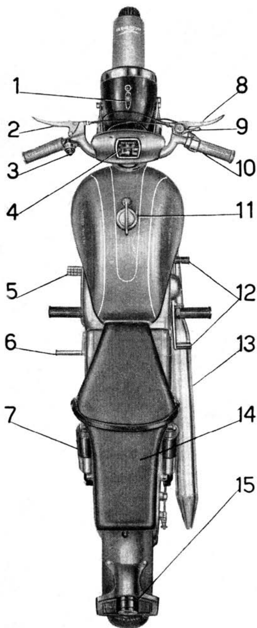
Fig. 5 - Comandi ed accessori
